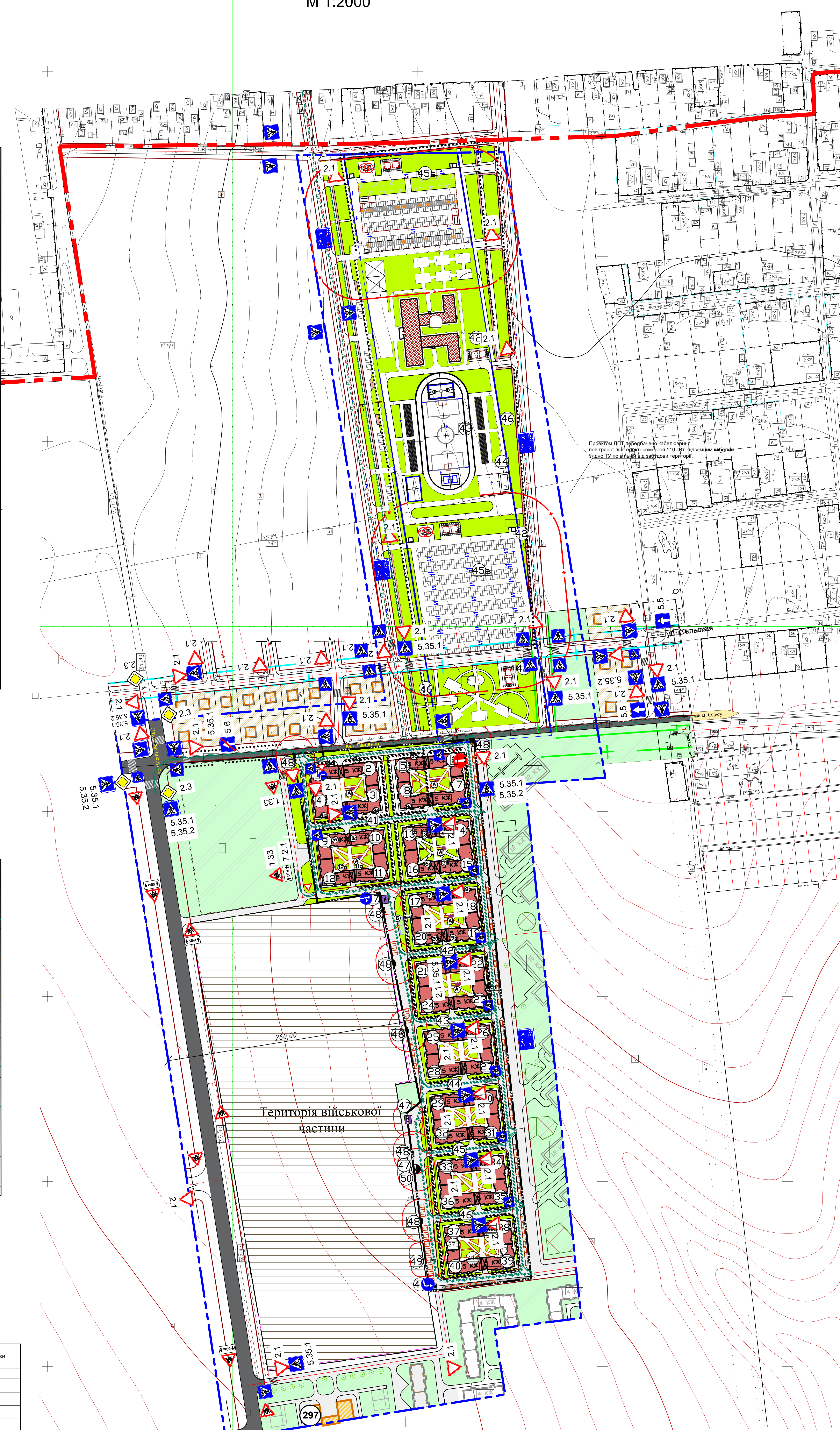
СХЕМА РУХУ ТРАНСПОРТУ ТА ПІШОХОДІВ М 1:2000
